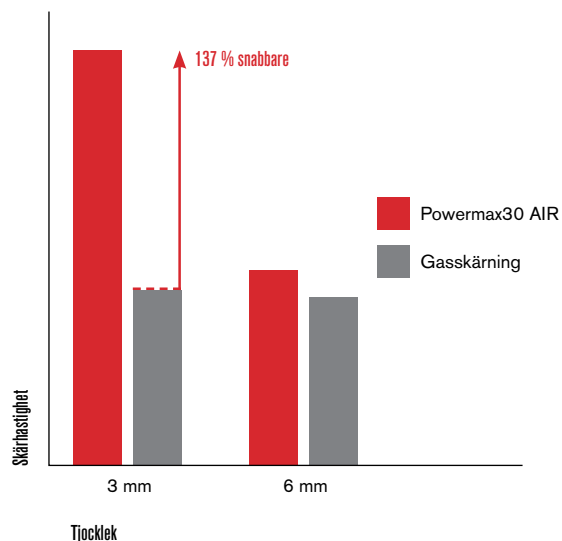
Relativ skärprestanda på mjukt kolstål
